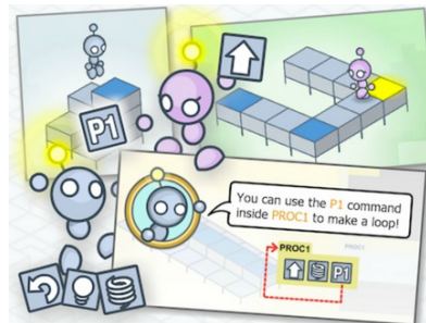
Lightbot
